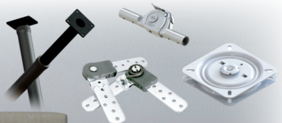
角度調整金具
