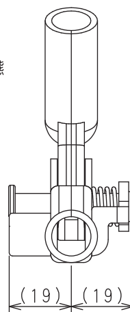
折曲げ状態
