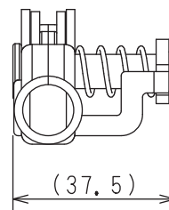
ロック状態
