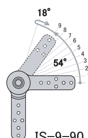
IS-9-90 zero position= 90° end position= 144°
